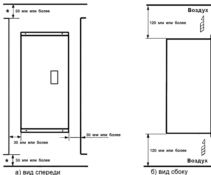
Рис. 3. Расстояния до окружающих устройств.
