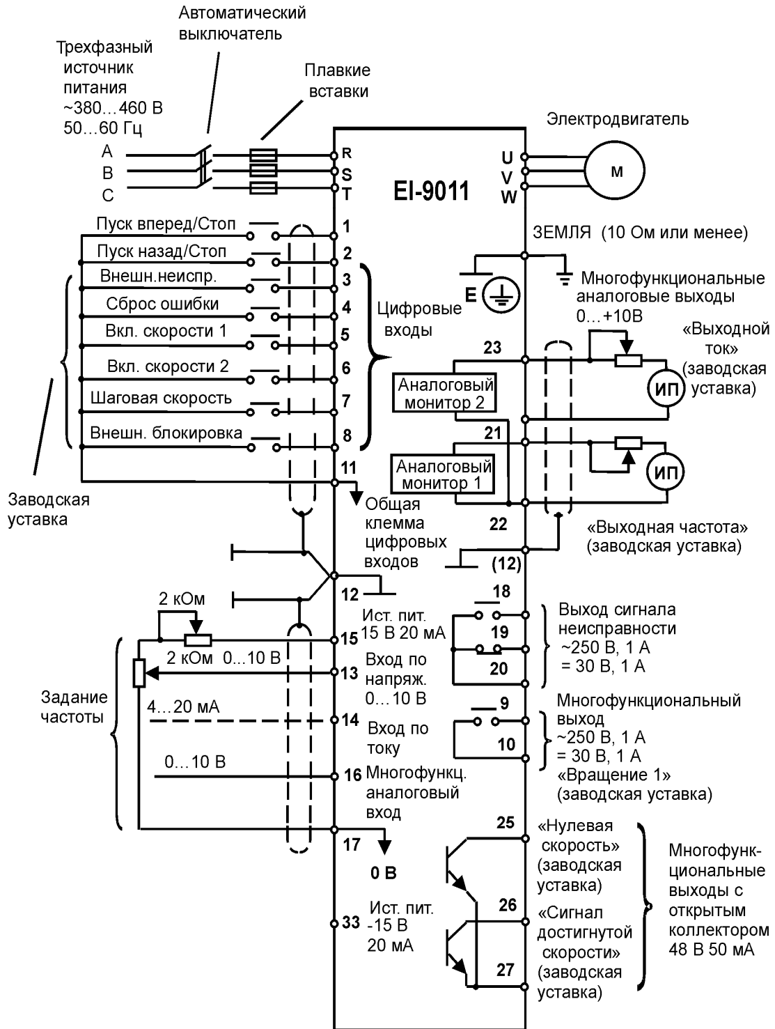
Рис. 4. Схема подсоединения
