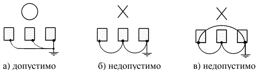
Рис. 10. Заземление нескольких преобразователей.
