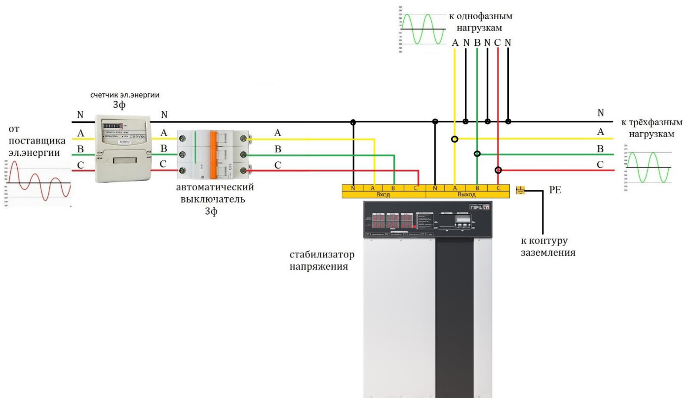
Рисунок 5. Схема подключения стабилизатора к трёхфазной сети
